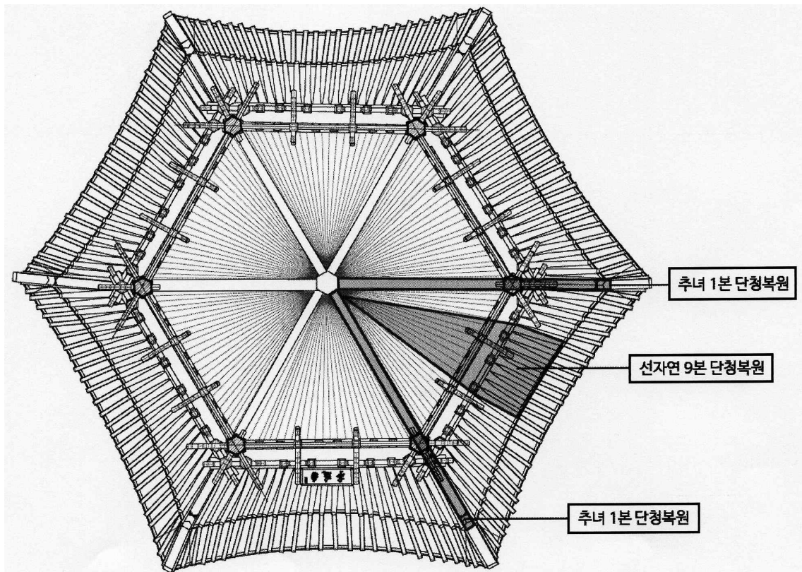
[천장 평면도]
