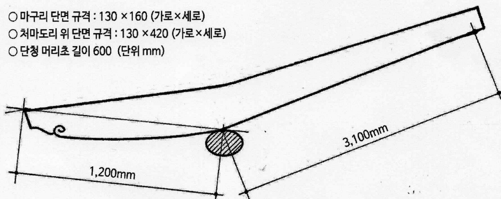
[추녀 상세도]
