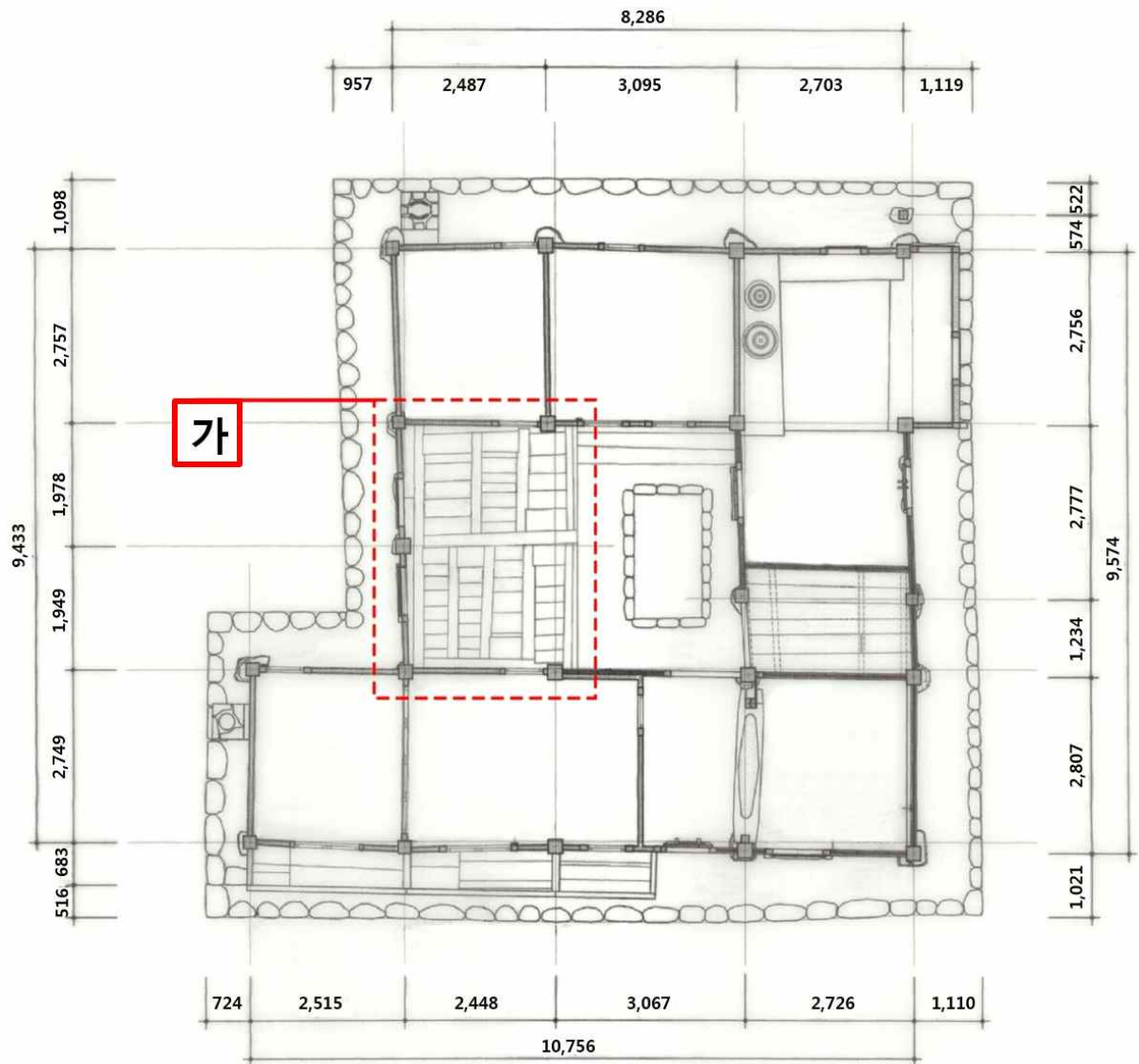
도면 1-1. 현황 실측 평면도
