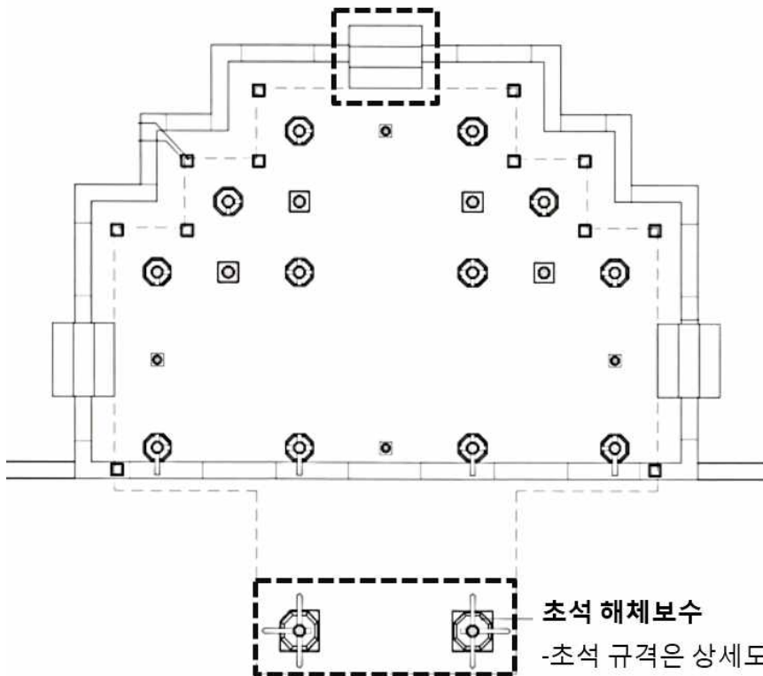
【 부용정 기단, 초석 평면도 】
